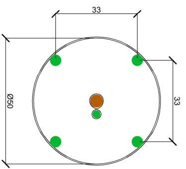
ELEVAÇÃO PLANTA
