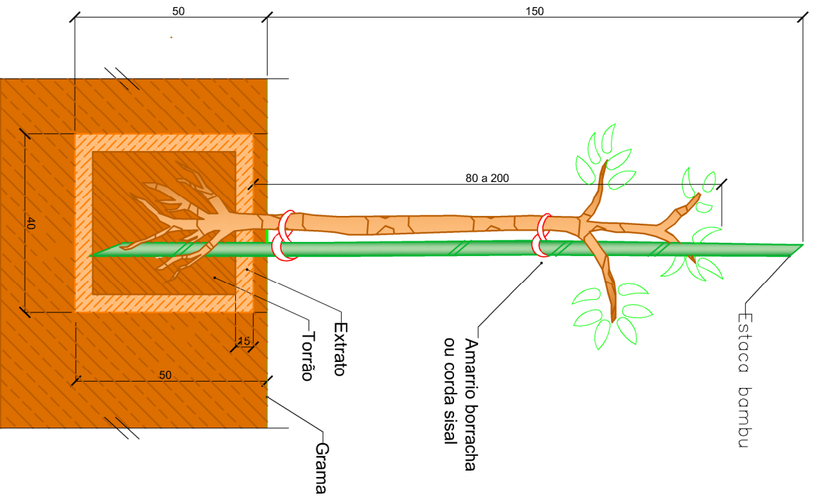
CORTE AA
