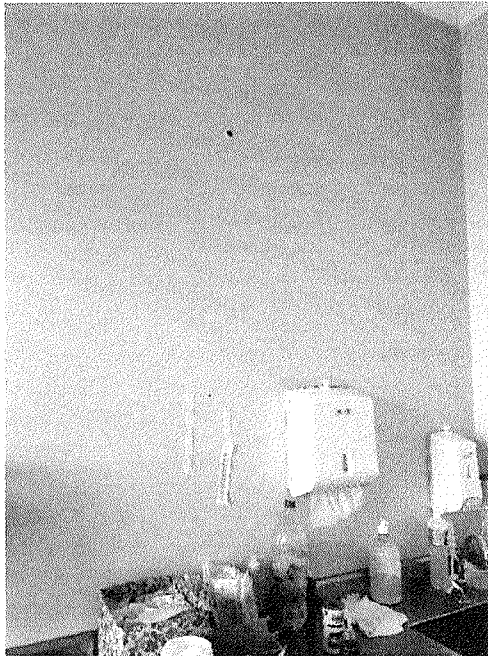
Figura 6 – Falta de vedação no orifício da tubulação hidrossanitária.
