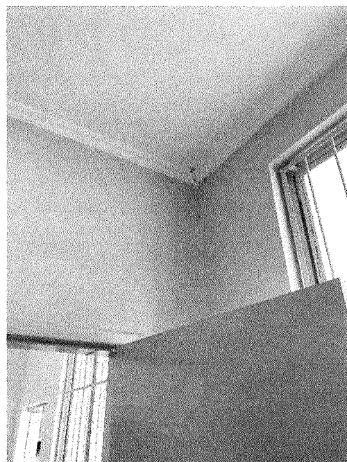
Figura 13 – Infiltração no orifício do cabo da sala de vacina.
