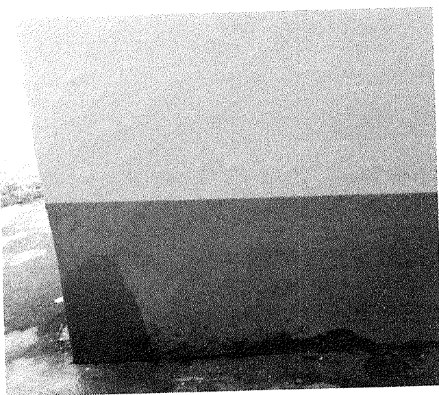
Figura 12 – Estufamento da pintura na parede externa da sala dos agentes de saúde.
