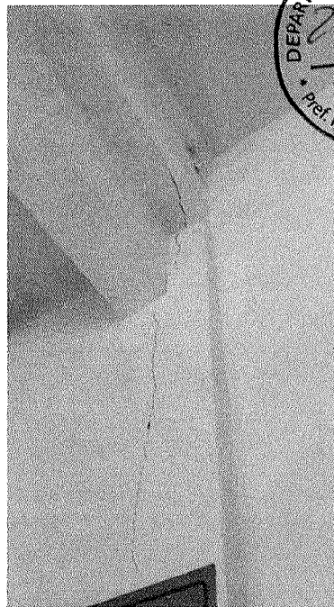
Figura 13 - Trinca
