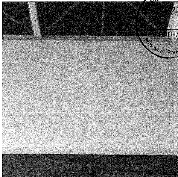
Figura 23 - Trinca na parede, cômodo 10
