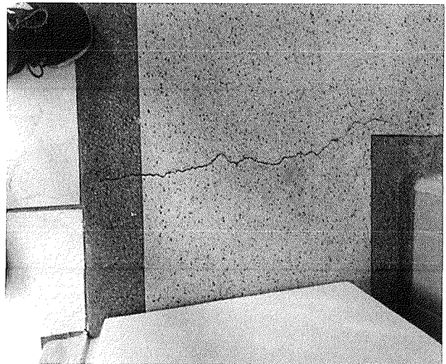
Figura 5 - Trinca no revestimento do banheiro 2
