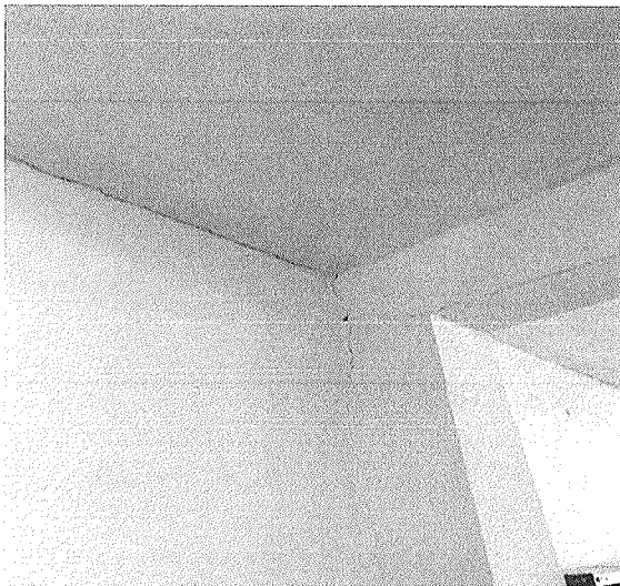
Figura 14 - Infiltração na laje
