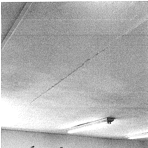
Figura 6 - Trinca na laje
