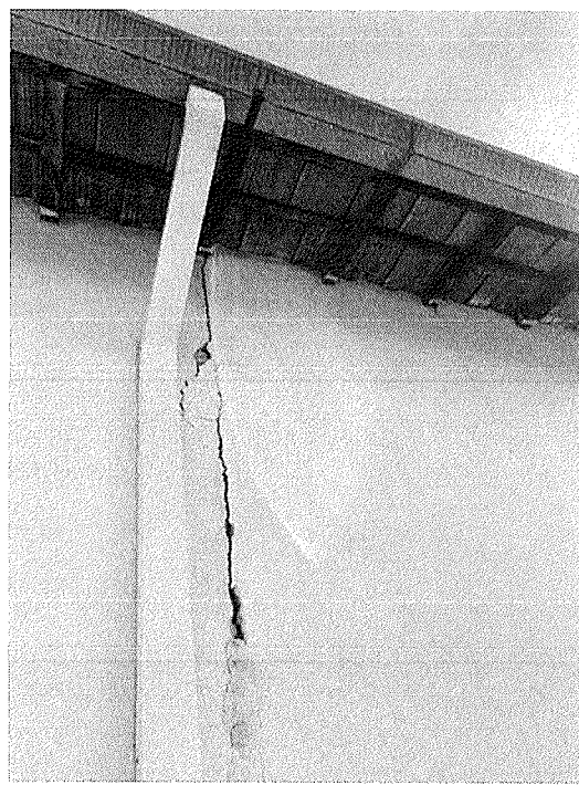
Figura 29 - Rachadura na parede
