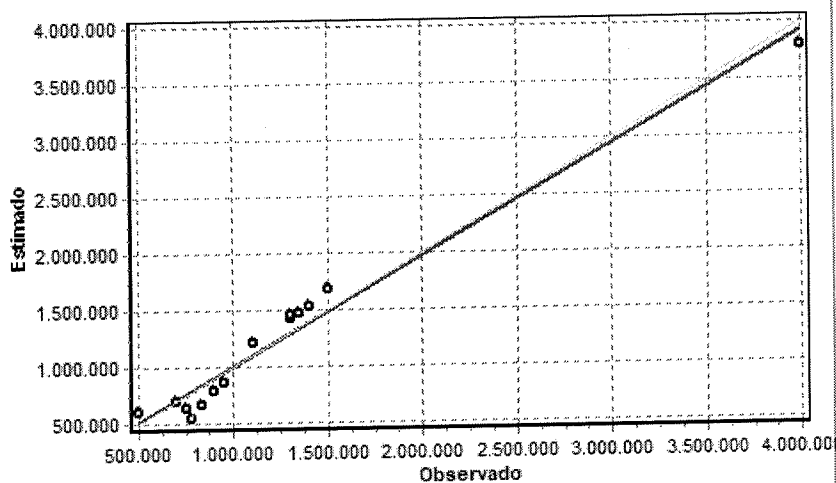
Gráfico de Aderência - Regressão Linear
